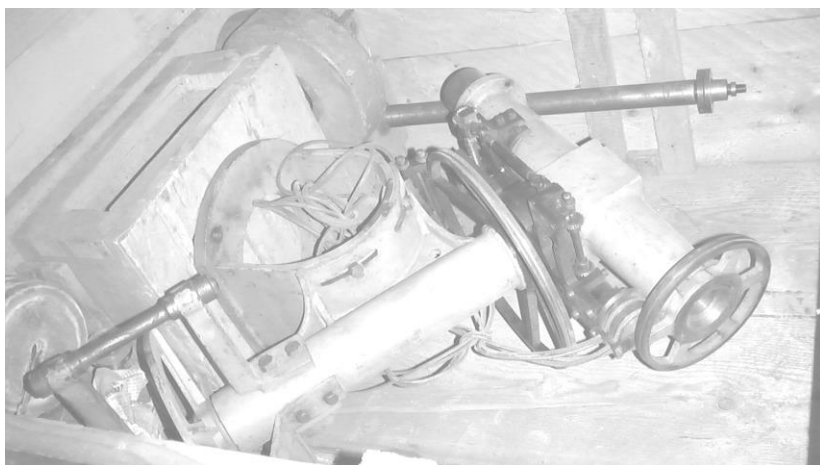
Ekvatorijalna montaža sa Zvezdarnice „Manora“
